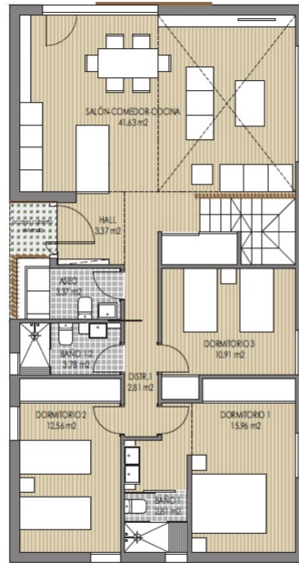
PLANTA BAJA
