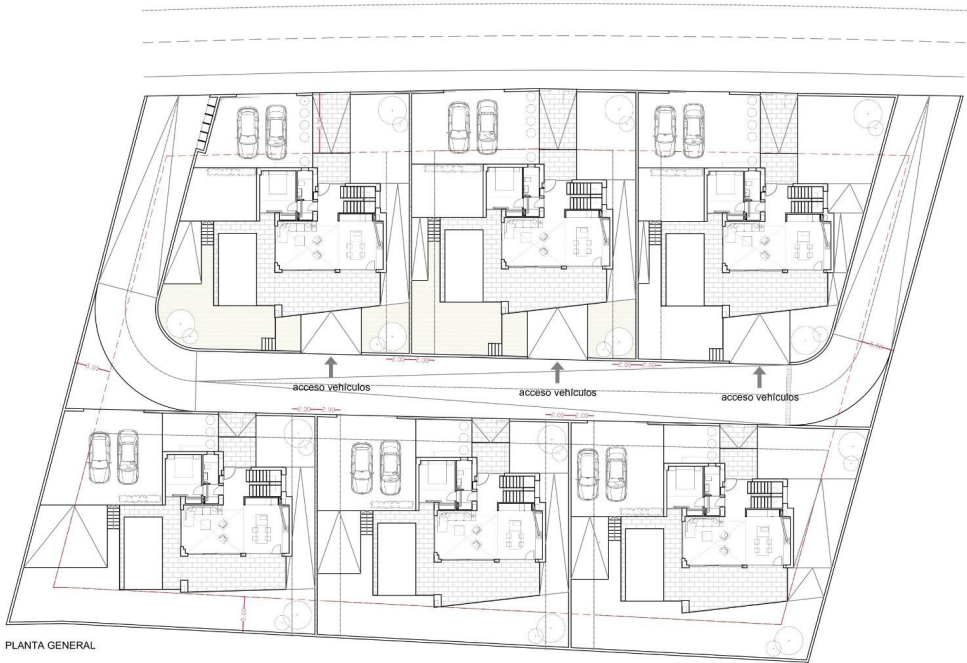
PLANTA GENERAL
