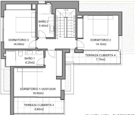
PLANTA ALTA - SUPERFICIES
