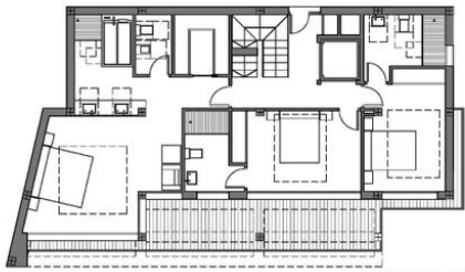
PLANTA PRIMERA
